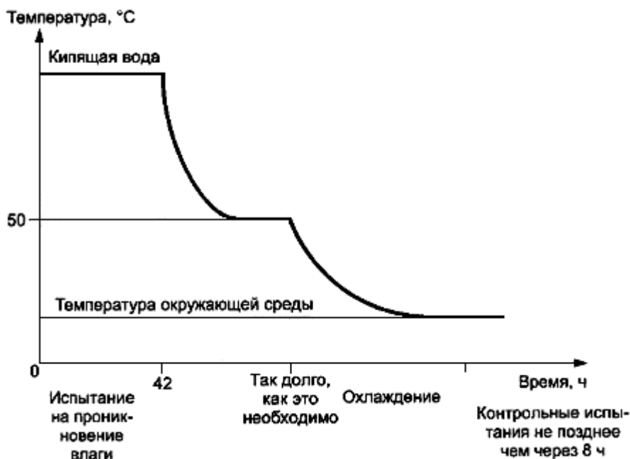
Рисунок 6 - Испытания на проникновение влаги
