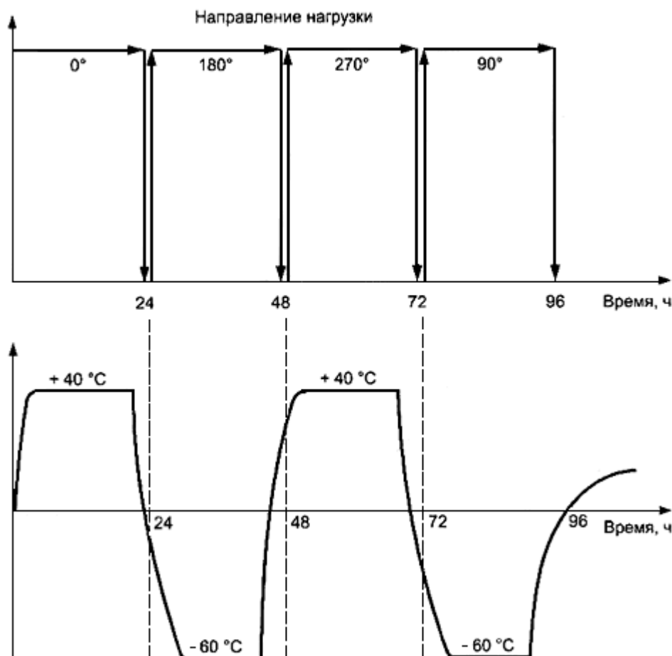
Рисунок 4 - Термомеханические испытания
