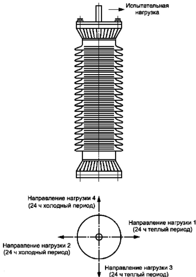
Рисунок 5 - Направления действия изгибающей нагрузки при термомеханических испытаниях
